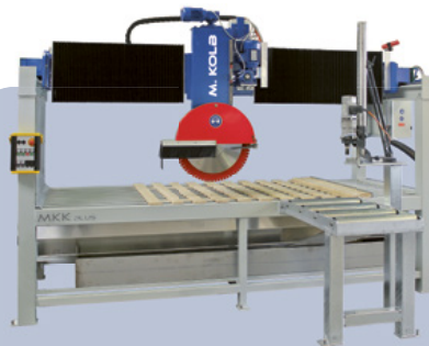
5-Achs-Technik für 3D Bearbeitung
