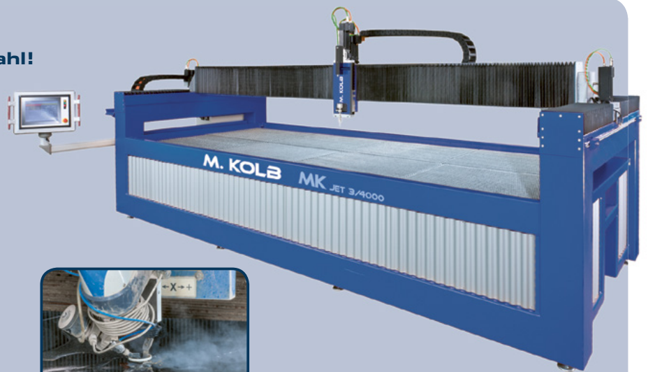
5-Achs-Technik für 3D Bearbeitung
